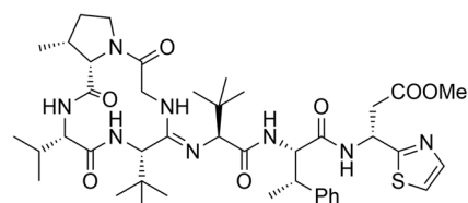
Fig. 1 Bottromycin A 2 .
