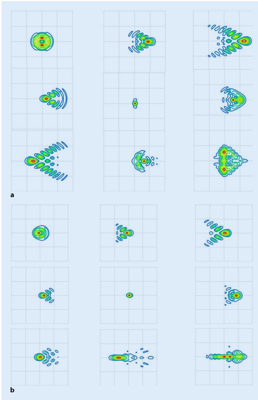
Abb. 4 ▲ a Punktbildverwaschungsfunktion („point spread function“) in der Bildebene für 9 ausgewählte Szenarien der Kombination aus Dezentrierung (in horizontale Richtung) und Verkippung (um die vertikale Achse) der natürlichen Augenlinse im Liou-Brennan-Modellauge bei einer Pupille mit 4 mm Durchmesser. Die linke/mittlere/rechte Spalte entsprechen einer Dezentrierung von -0,6/0,0/0,6 mm, die obere/mittlere/untere Reihe einer Verkippung um 6/0/-6^\circ . Jede Skalenteilung in horizontale und vertikale Richtung hat eine Abmessung von 10\ \mu\text{m} in der Bildebene. b Punktbildverwaschungsfunktion („point spread function“) in der Bildebene für 9 ausgewählte Szenarien der Kombination aus Dezentrierung (in horizontale Richtung) und Verkippung (um die vertikale Achse) der Kunstlinse (Z9000) als Ersatz der natürlichen Linse im Liou-Brennan-Modellauge bei einer Pupille mit 4 mm Durchmesser. Die linke/mittlere/rechte Spalte entsprechen einer Dezentrierung von -0,6/0,0/0,6 mm, die obere/mittlere/untere Reihe einer Verkippung um 6/0/-6^\circ . Jede Skalenteilung in horizontale und vertikale Richtung hat eine Abmessung von 10\ \mu\text{m} in der Bildebene
