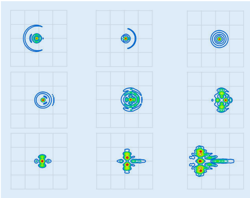
Abb. 5 ▲ Punktbildverwaschungsfunktion („point spread function“) in der Bildebene für 9 ausgewählte Szenarien der Kombination aus Dezentrierung (in horizontale Richtung) und Verkippung (um die vertikale Achse) für eine sphärische equikonvexe Kunstlinse (hier wurden die gleichen Materialeigenschaften und der gleiche Brechwert von 21 dpt wie bei der Z9000 angenommen) als Ersatz der natürlichen Linse im Liou-Brennan-Modellauge bei einer Pupille mit 4 mm Durchmesser. Die linke/mittlere/rechte Spalte entsprechen einer Dezentrierung von -0,6/0,0/0,6 mm, die obere/mittlere/untere Reihe einer Verkippung um 6/0/-6^\circ . Jede Skalenunterteilung in horizontale und vertikale Richtung hat eine Abmessung von 10\ \mu\text{m} in der Bildebene
