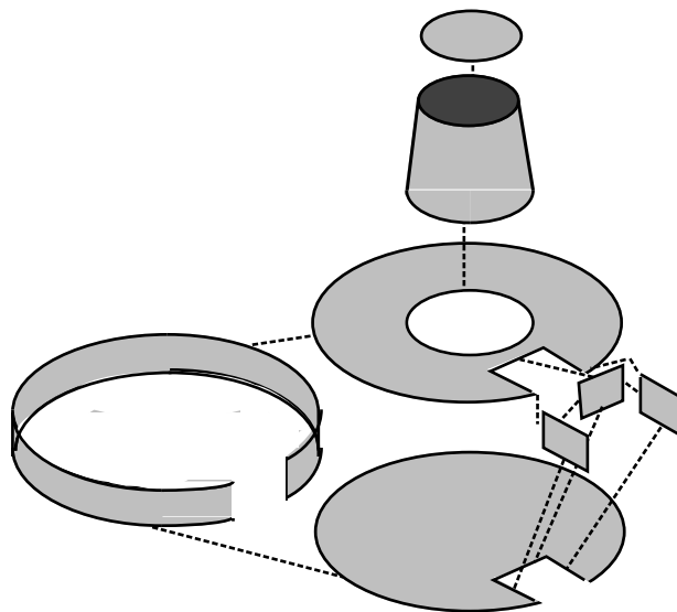
Der gleiche Gegenstand in BREP-Darstellung
