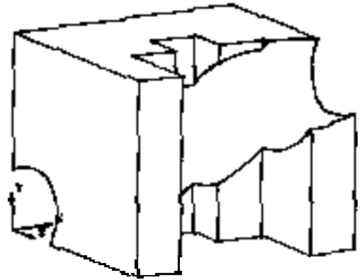
Subtraktion A \setminus B
