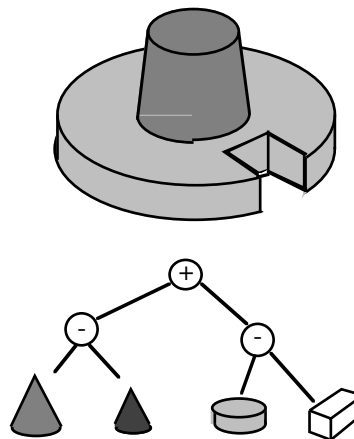
CSG-Darstellung eines Werkstücks
