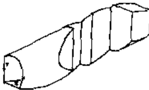
Durschnitt A \cap B
